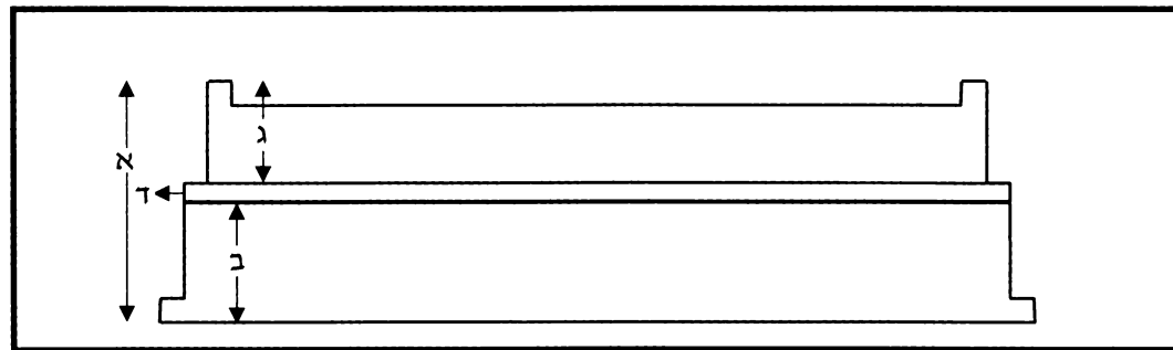
814. מזבח כמה הוה ליה שיתין [א], פלגיה דמזבח כמה הוה תלתין [ב], מקרנות ועד סובב כמה הוי כ"ד [ג], כמה בציר לפלגיה דמזבח ששה [ד], ותנן אם עשאה למטה מרגליו אפילו אמה אחת כשרה.
