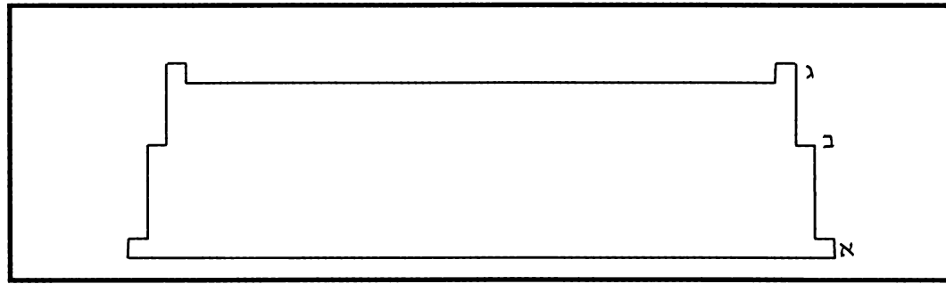
813. רשיי ד"ה אלא, כולה עשר אמות דגובה המזבח באמה בת ששה, וכי קתני באמה בת חמש באמות דכניסה יסוד [א] וסובב [ב] ועובי הקרנות [ג].
